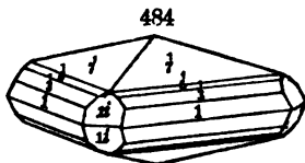
Binnenthal.
